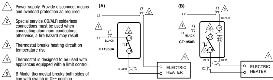
Fig. 1 Wiring
